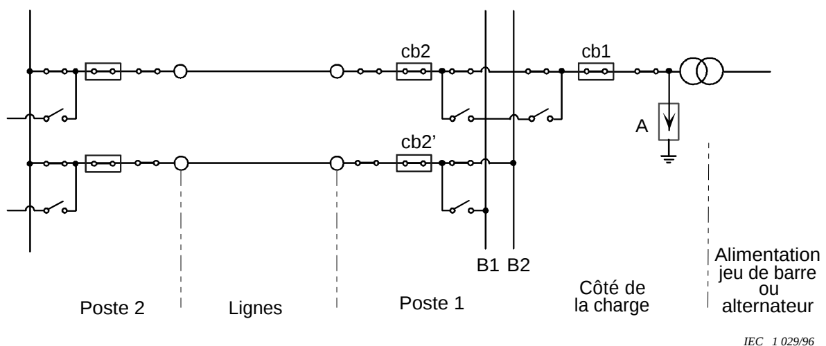
Figure 11 – Exemple de disposition schématique de poste utilisé pour la localisation des contraintes (voir 7.1)
