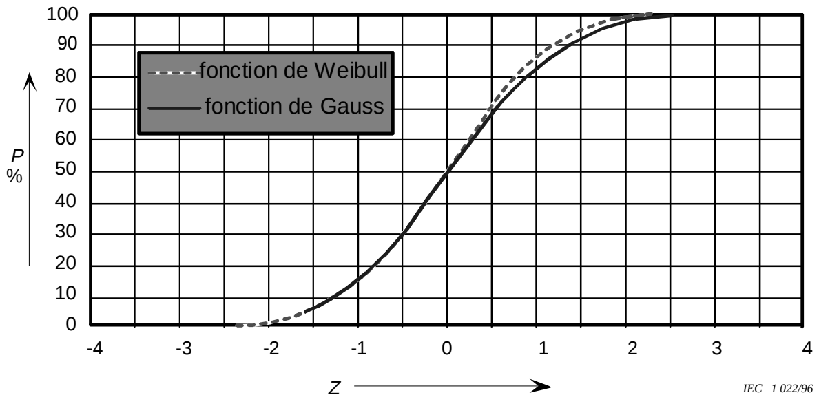
Figure 4 – Probabilité de décharge disruptive d'une isolation autorégénératrice sur une échelle linéaire
