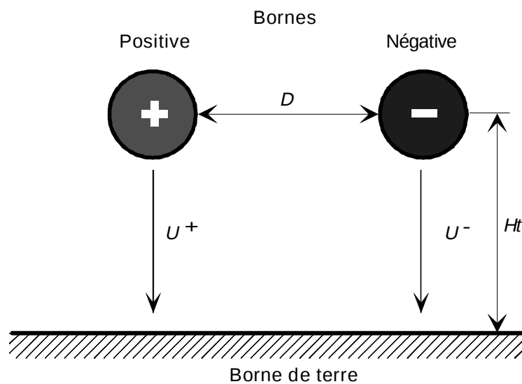
Figure D.2 – Principe de détermination de la surtension représentative entre phases U_{pre}
